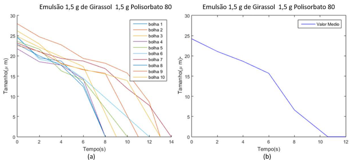
Figura 47 - Curva de estabilidade da população de microbolhas para emulsão de água, óleo de girassol e polissorbato 80 (97: 1,5: 1,5).
