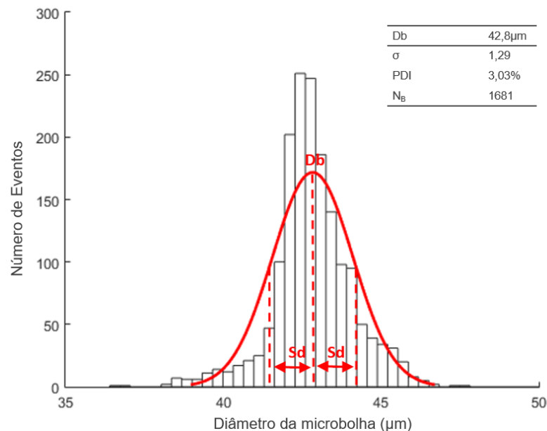
Figura 44 - Curva de distribuição do segundo experimento de microbolhas geradas em elevada taxa de produção.
