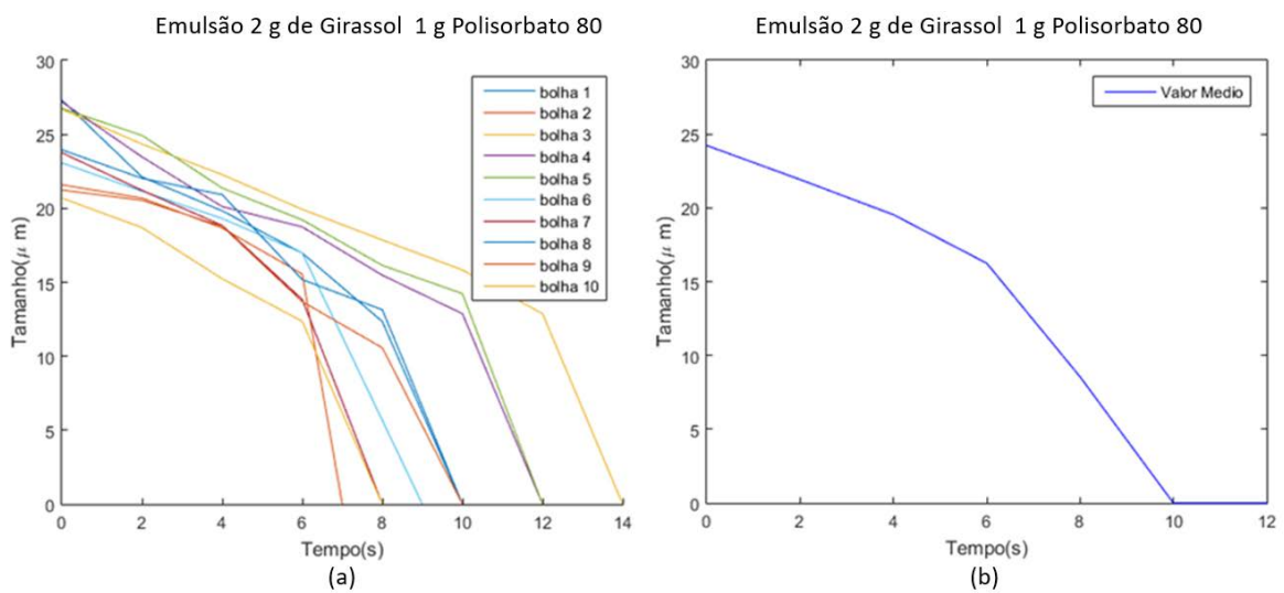
Figura 46 - Curva de estabilidade da população de microbolhas para emulsão de água, óleo de girassol e polissorbato 80 (97: 2: 1).
