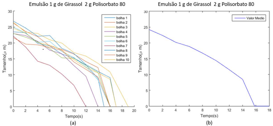
Figura 48 - Curva de estabilidade da população de microbolhas para emulsão de água, óleo de girassol e polissorbato 80 (97: 1: 2).
